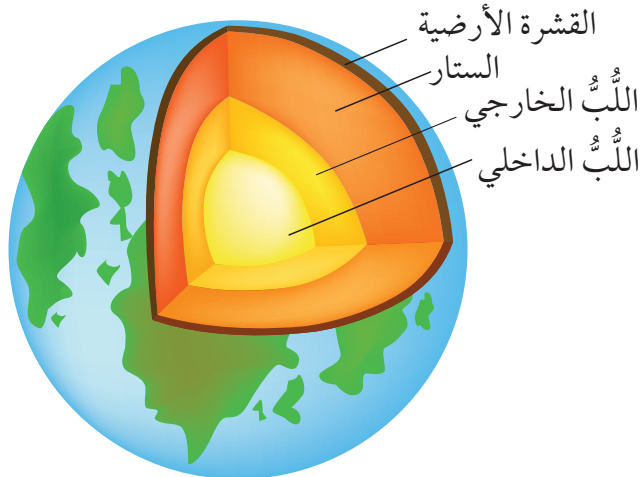
الشكل (2): النُطُق الرئيسية للأرض وتمايزها بعد تشكّل الأرض.
