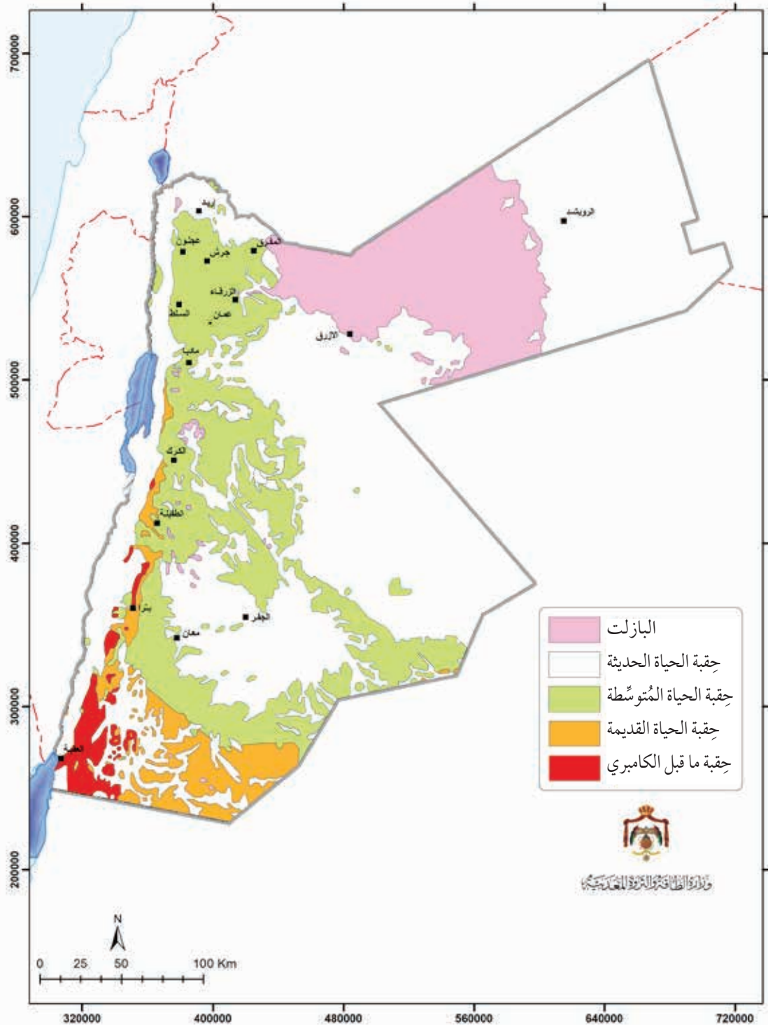
الشكل (33): خريطة توزع الصخور في الأردن بحسب الحقب التي تتبع لها. أحدّد: أين تتكشف صخور حِقبة ما قبل الكامبري في الأردن؟
